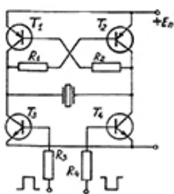
Рис.21. Мостовая схема оконечного устройства питаемая повышенным (десятки вольт) напряжением. Транзисторы: Т1,Т2 - КТ-502Г, КТ-973А, КТ-8147А Т3,Т4 - КТ-503Г, КТ-972А, КТ-8116А Резисторы R1 – R4 5 – 10 кОм.
