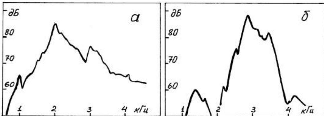
Рис.5. а) Частотная характеристика широкополосного звонка ПВА-1;
