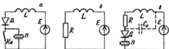
Рис.16. а) Упрощённая схема окончного устройства; б) эквивалентная схема для полупериода с замкнутым ключём; в) эквивалентная схема для полупериода с разомкнутым ключём.
